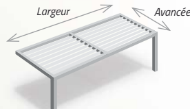
Pergola deux modules, lames parallèles à la façade Avancée jusqu'à 5560 mm Largeur jusqu'à 7500 mm A partir de 3840 mm d'avancée et/ou 6000 mm de largeur, un poteau intermédiaire est ajouté pour assurer un parfait maintien de la structure
