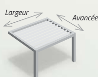
Pergola un module, lames parallèles à la façade Avancée jusqu'à 5910 mm Largeur jusqu'à 4000 mm
