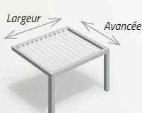
Pergola un module, lames perpendiculaires à la façade Avancée jusqu'à 4000 mm Largeur jusqu'à 5910 mm
