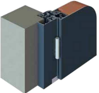
POSE EN FEUILLURE Dormant large sans aile + compensateur de feuillure
